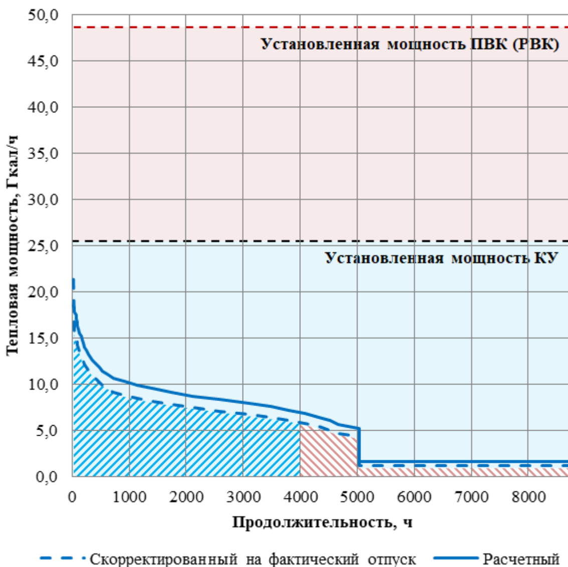
Рисунок 17 – График Россандера для ГТУ-ТЭЦ за 2017 год
