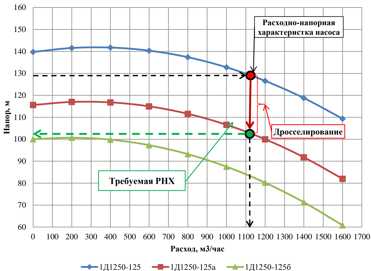
Рисунок 13 – Расходно-напорная характеристика насоса 1Д-1250-125
