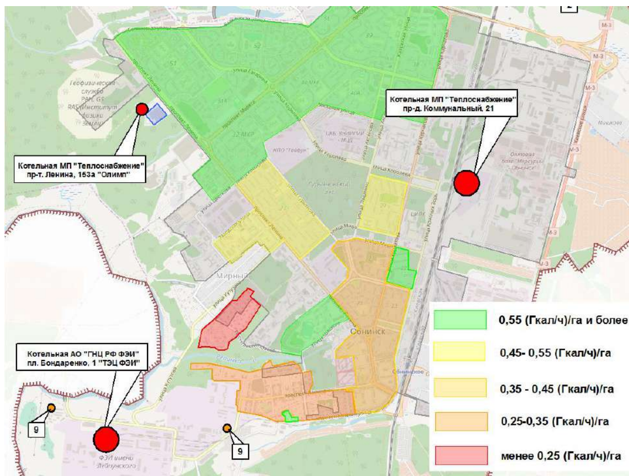
Рисунок 31 - Плотность нагрузок в зоне действия городской котельной МП «Теплоснабжение» и ТЭЦ ФЭИ
