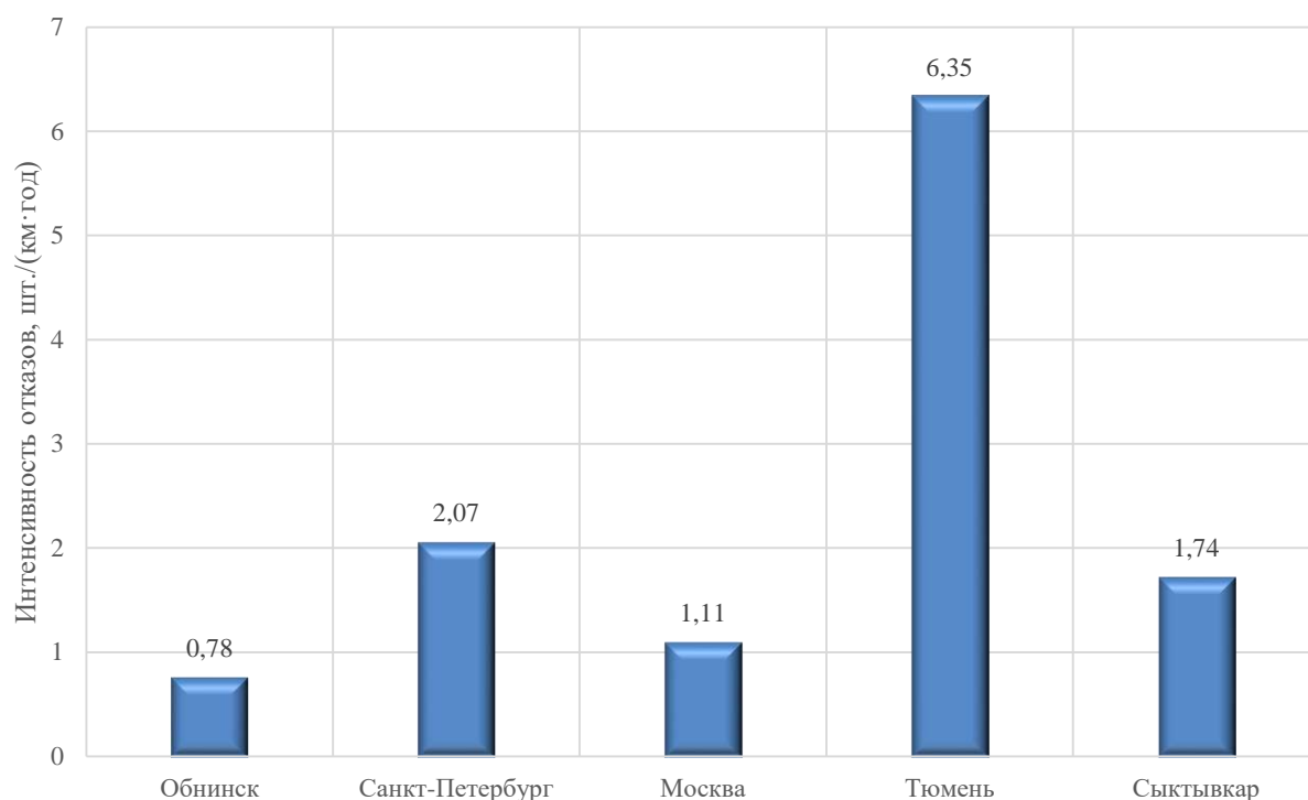
Рисунок 29 - Сравнение показателя интенсивности отказов тепловых сетей по МП «Теплоснабжение» с аналогичным показателем для других городов
