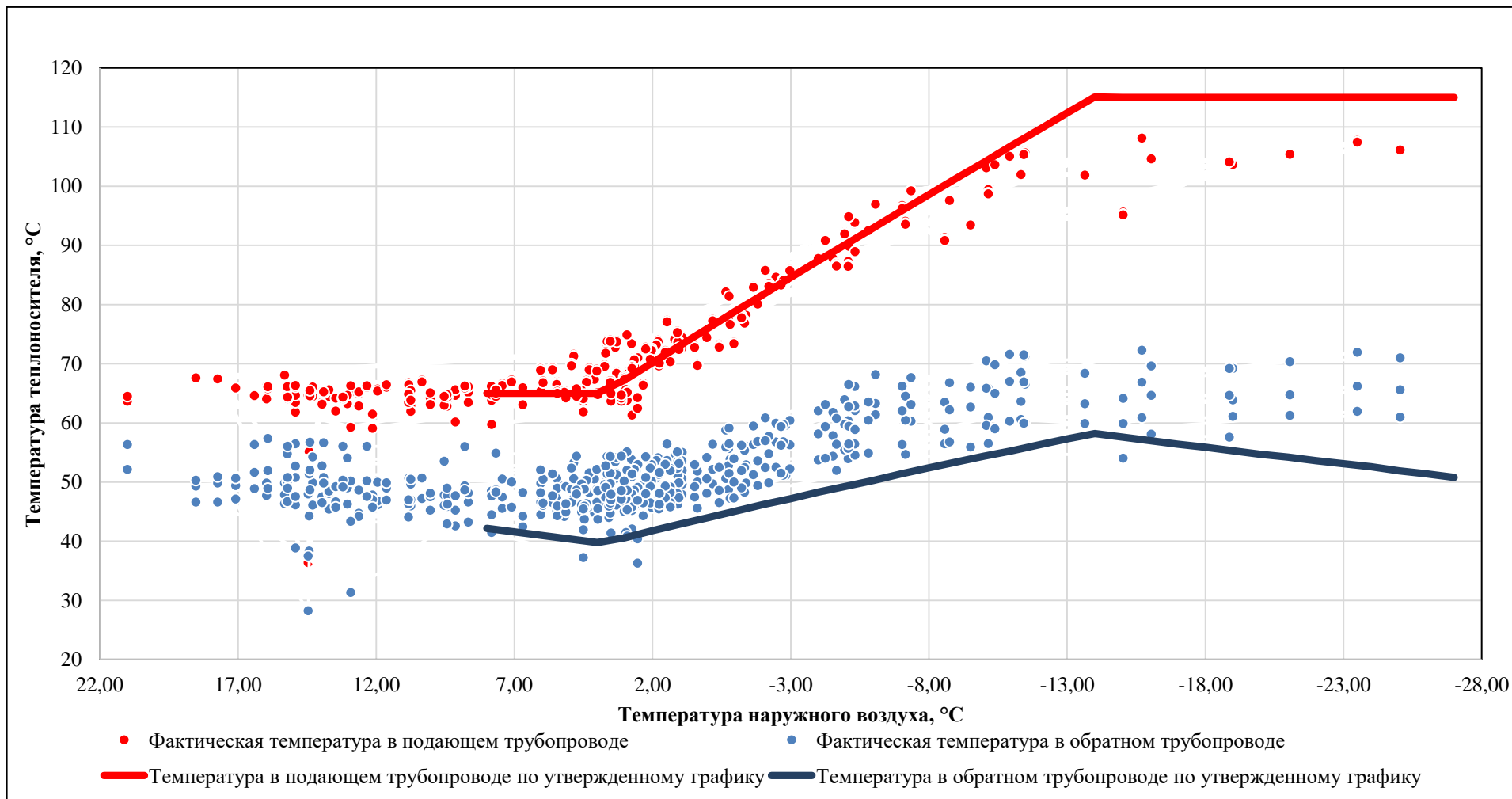
Рисунок 20 – Сравнение фактического и утвержденного температурных графиков ТЭЦ ФЭИ (150/70°С со срезкой на 115°С и изломом на 65°С)
