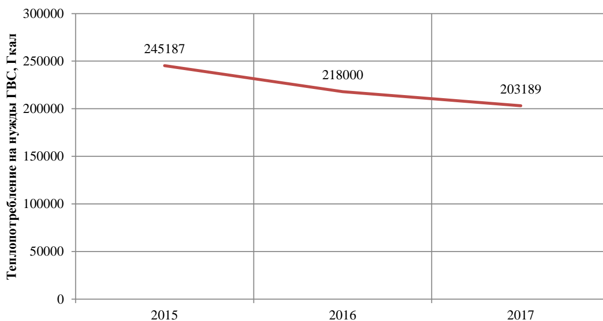
Рисунок 28 - Динамика потребления тепловой энергии на нужды ГВС абонентами котельной по адресу: Коммунальный пр., 21
