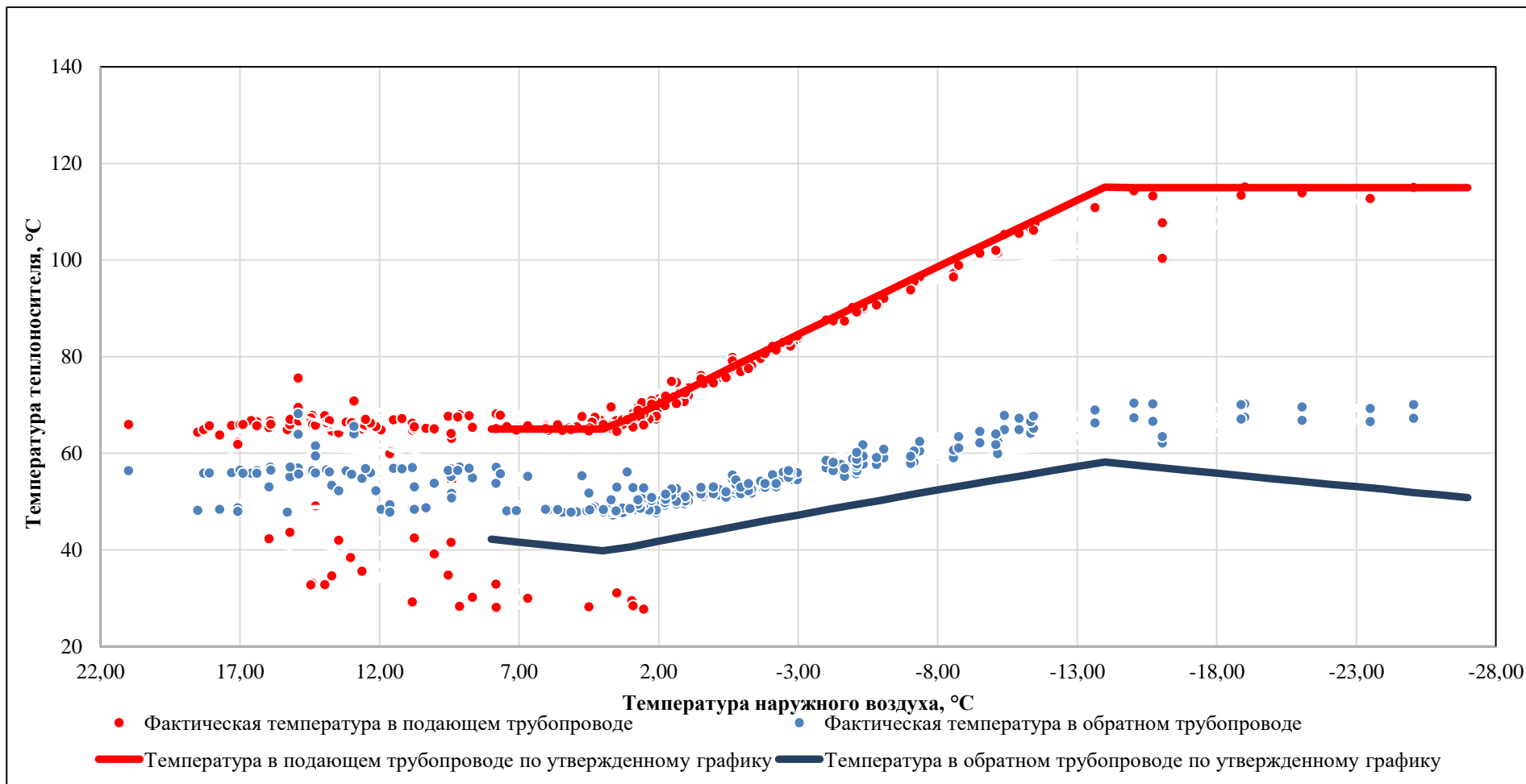
Рисунок 19 - Сравнение фактического и утвержденного температурных графиков котельной МП «Теплоснабжение» (150/70°C со срезкой на 115°C и изломом на 65°C)
