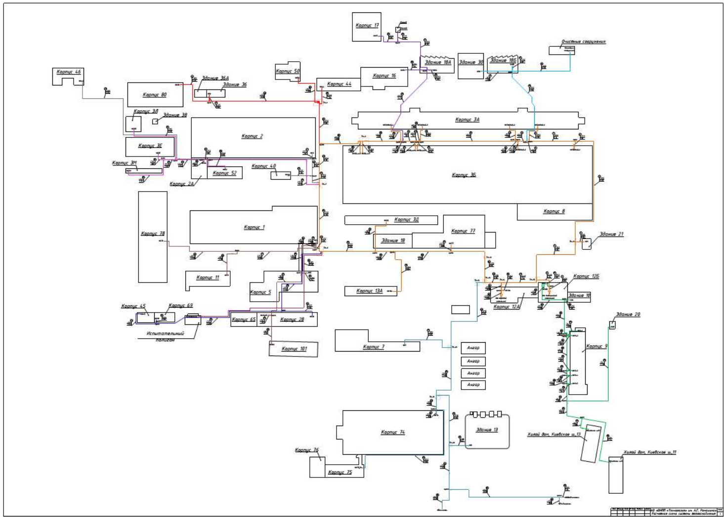
Рисунок 12 - Тепловые сети от котельной АО «ОНПП «Технология» им. А. Г. Ромашина»
