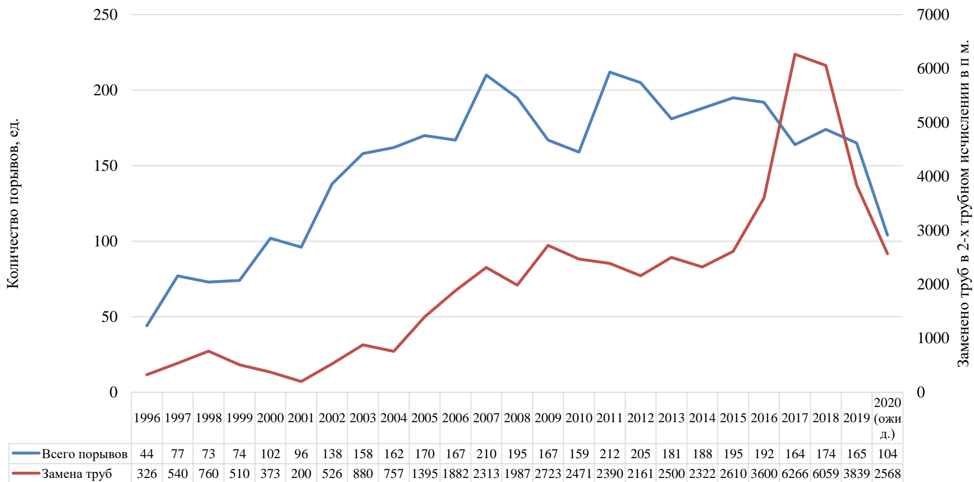
Рисунок 22 - Соотношение количества порывов на тепловых сетях с объемами их ремонтов по зоне действия МП «Теплоснабжение» и ТЭЦ ФЭИ
