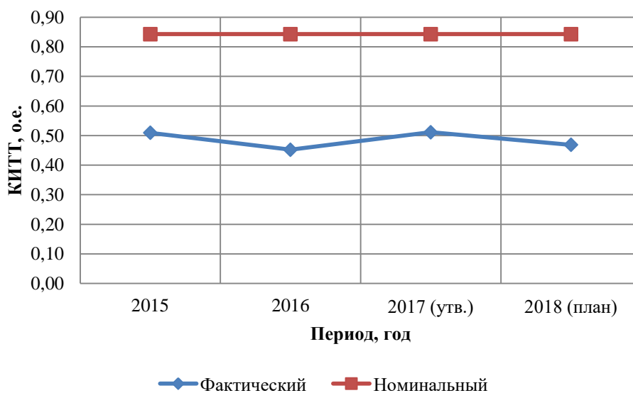
Рисунок 34 - Коэффициент использования тепла топлива
