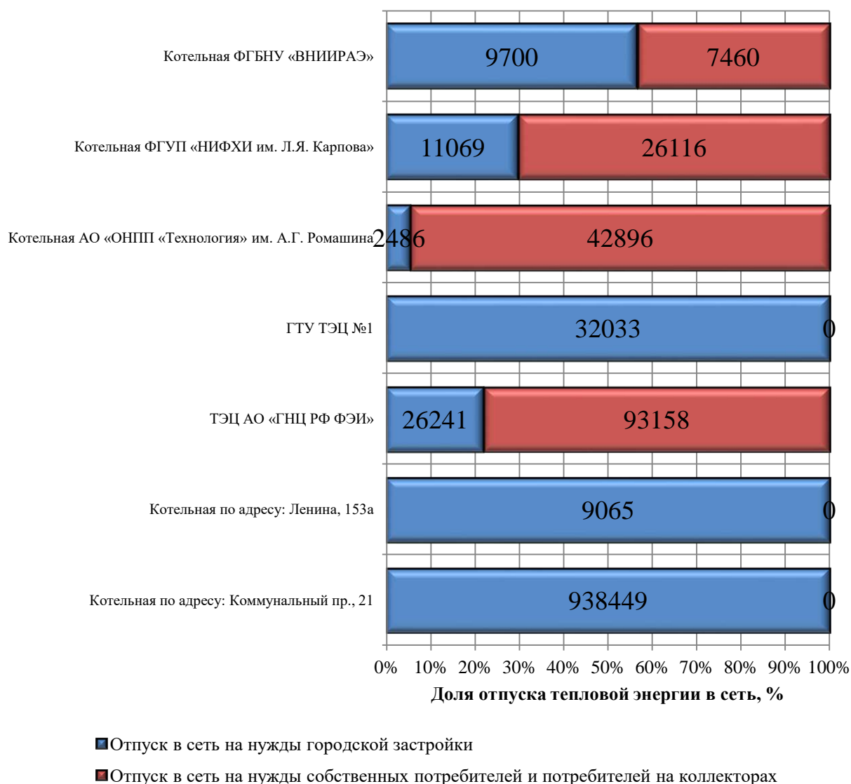
Рисунок 25 - Структура отпуска тепловой энергии в сеть по группам потребителей за 2016 г.
