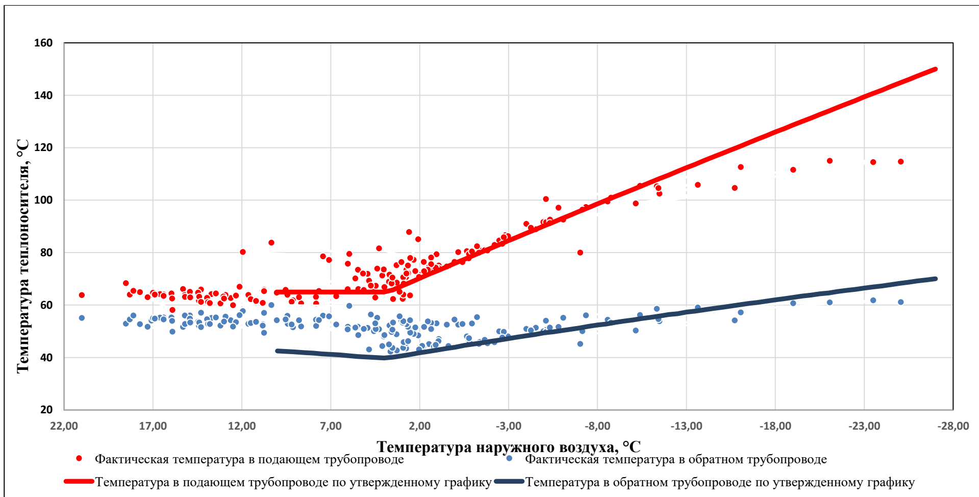
Рисунок 21 – Сравнение фактического и утвержденного температурных графиков ГТУ ТЭЦ (150/70°С с изломом на 65°С)
