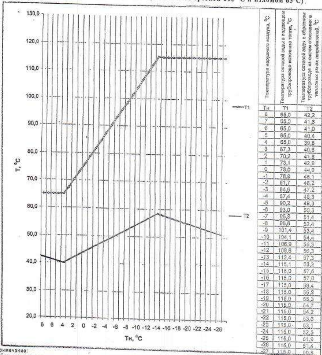
Расчетный график температуры воды для тепловой сети МП «Теплоснабжение» в отопительном сезоне 2017-2018г.г. (150-70°C со срезкой 115° С и изломом 65°С).
