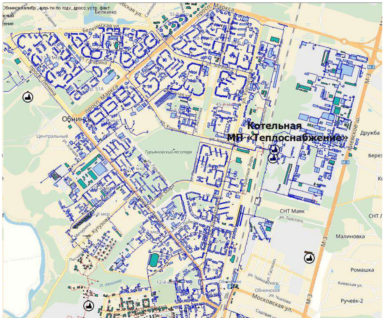
Рисунок 7 – Тепловые сети от котельной МП «Теплоснабжение»
