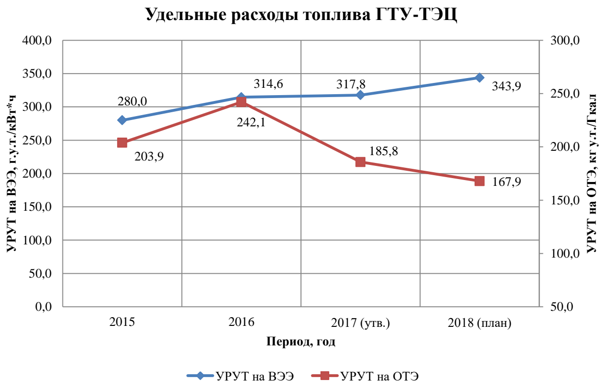
Рисунок 33 - Удельные расходы топлива ГТУ-ТЭЦ
