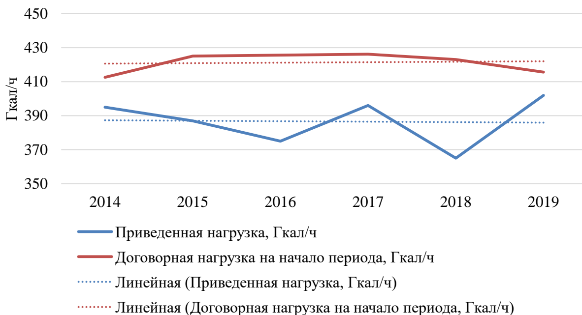
Рисунок 27 - Динамика изменения приведенной и договорной нагрузки по МП «Теплоснабжение»
