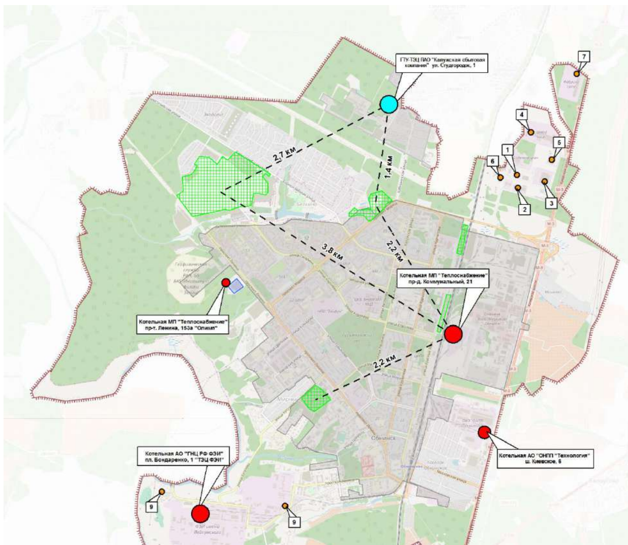
Рисунок 32 - Перспективные зоны централизованного теплоснабжения
