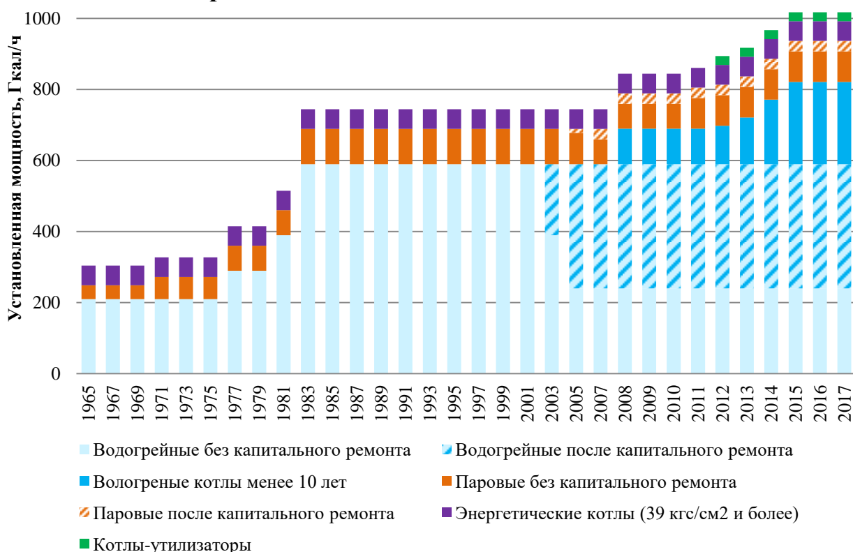
Рисунок 3 - Состав и срок ввода тепловой мощности источников централизованного теплоснабжения г. Обнинск
