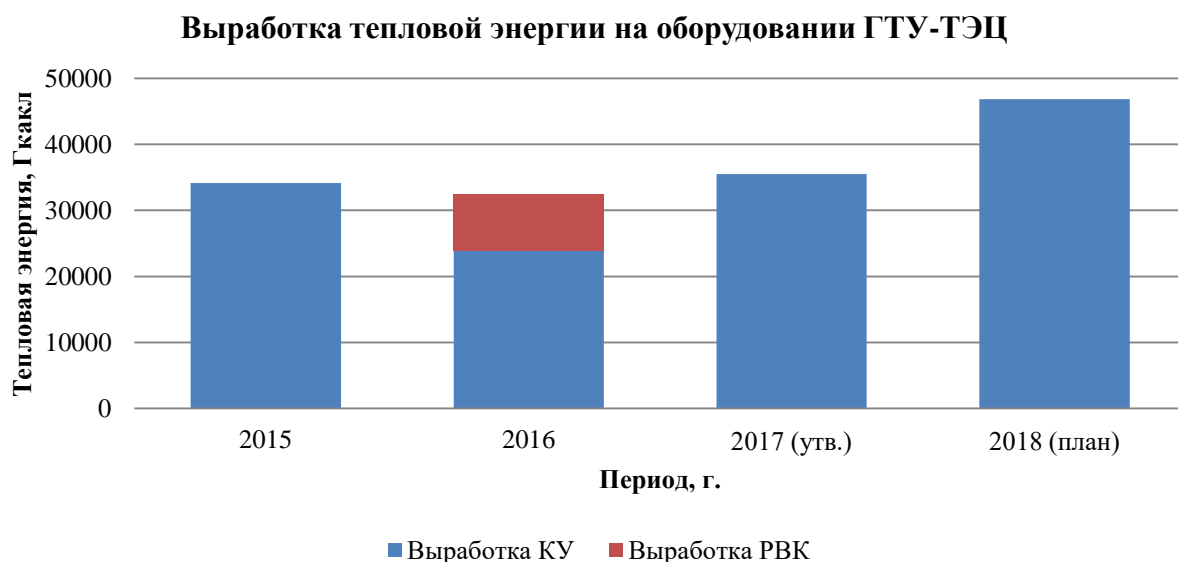
Рисунок 5 – Балансы выработки тепловой энергии на оборудовании ГТУ-ТЭЦ
