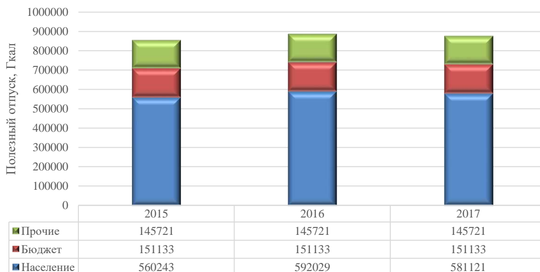
Рисунок 26 - Структура полезного отпуска тепловой энергии потребителям МП «Теплоснабжение»
